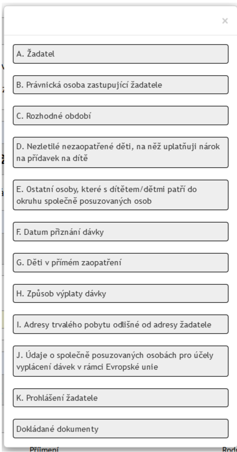
Obrázek 15: Navigační menu
